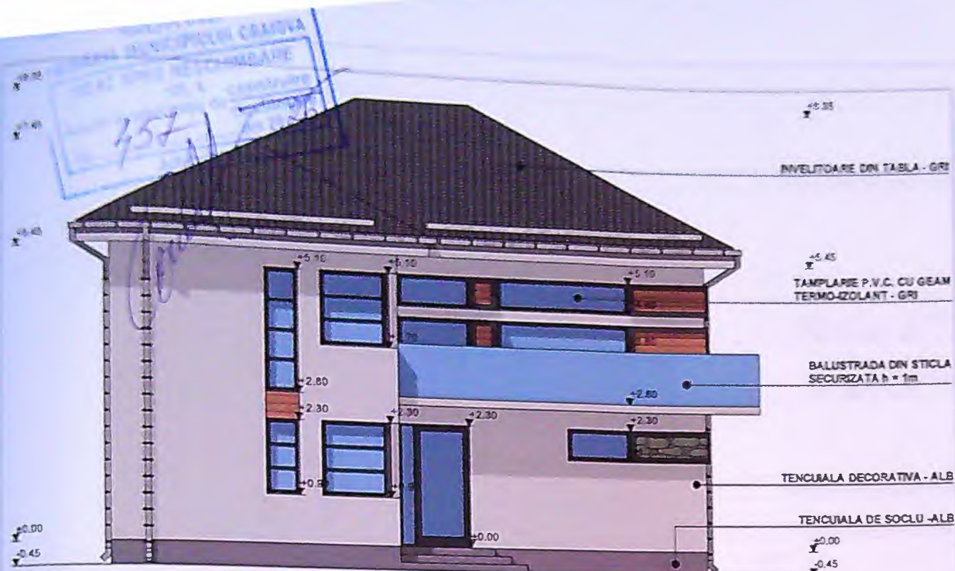
FATADA SUD
